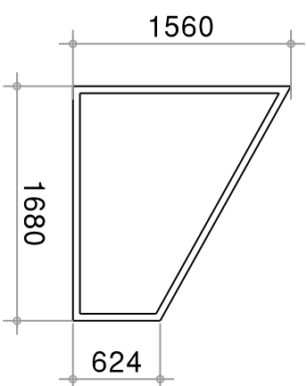
О-9 (1 шт)
